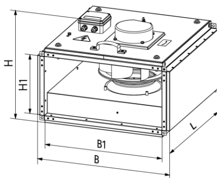
Box-I EC 30x15 - Box-I EC 60x30
