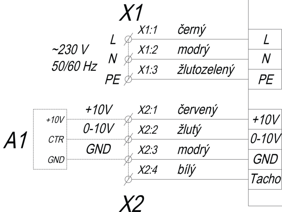
Zapojení Box EC, jednofázové
