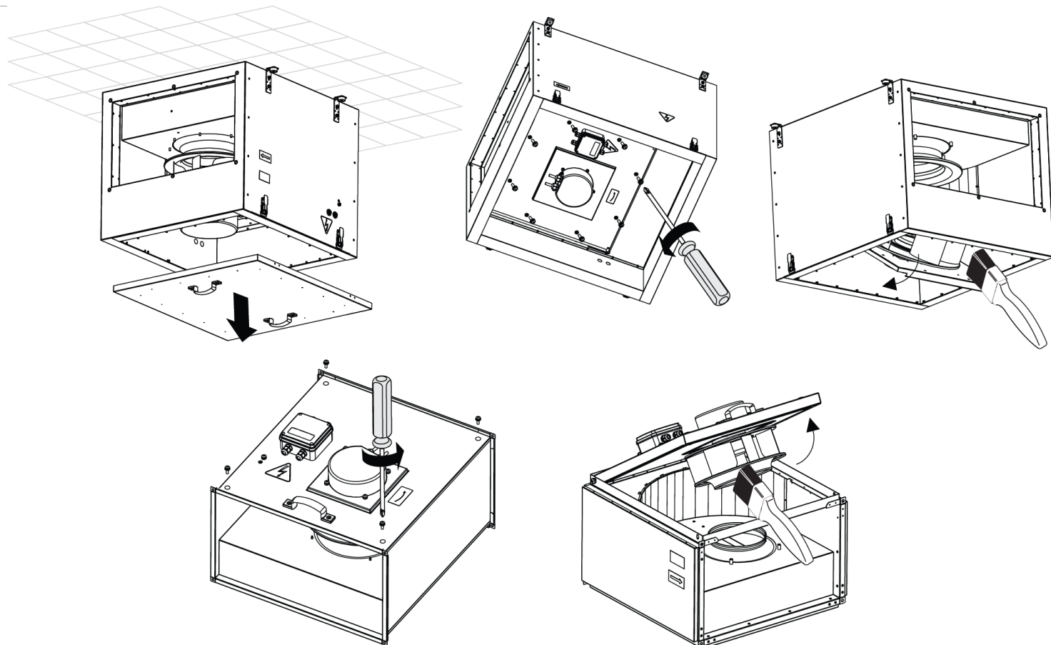
Box-I EC Servis
