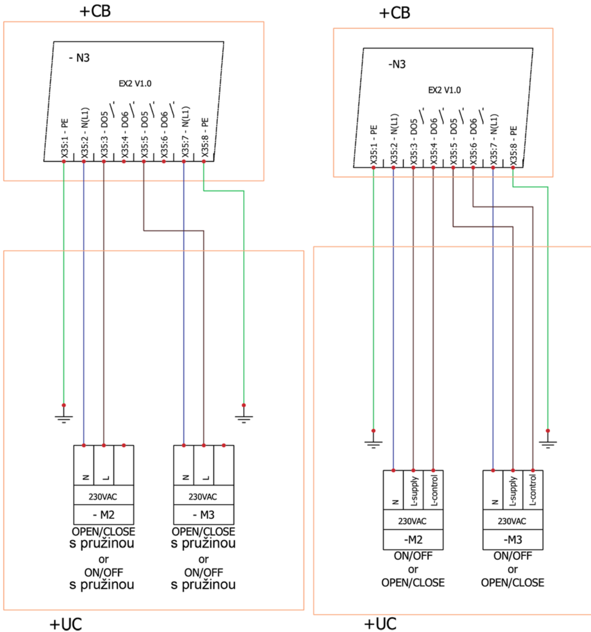
Klapky s servopohon
