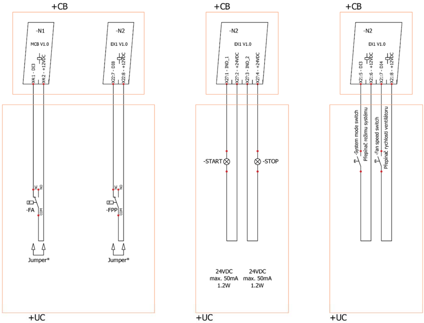
Kontakt požárního poplachu
