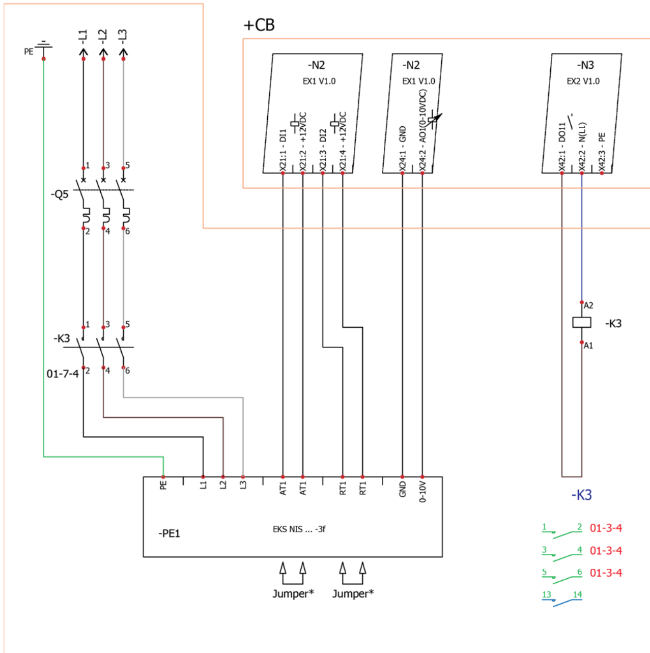
Elektrický externí předešřivač
