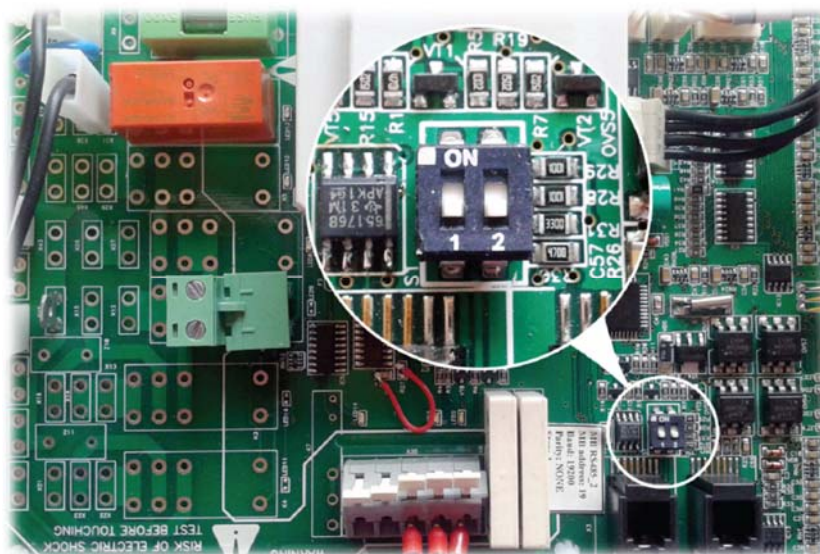
Mikrospínače 1 a 2
